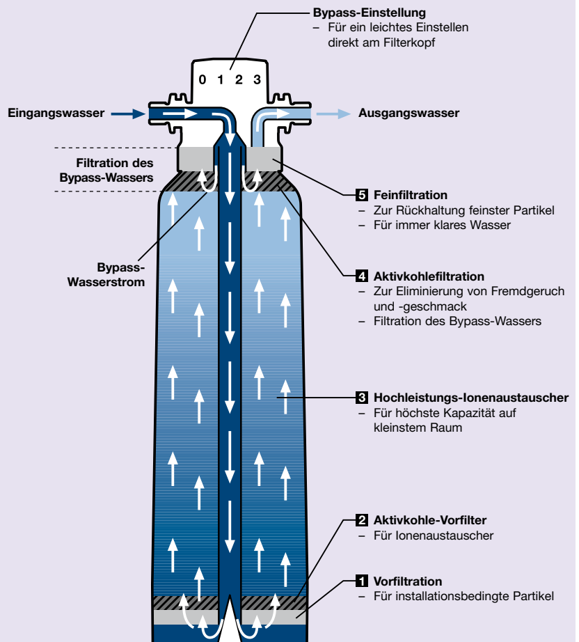
Aufbau einer bestprotect-Filterkerze mit 5-fach-Filtration
